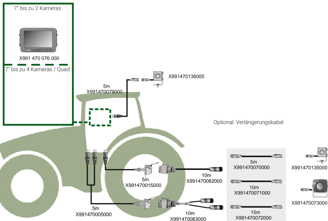
Kamera X991470073000
