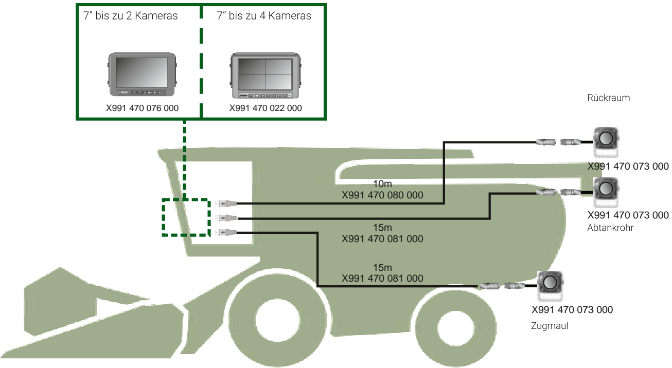
Rückfahrkamera X991470073000
