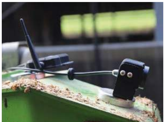
Magnetfuß-Befestigung Kamera
